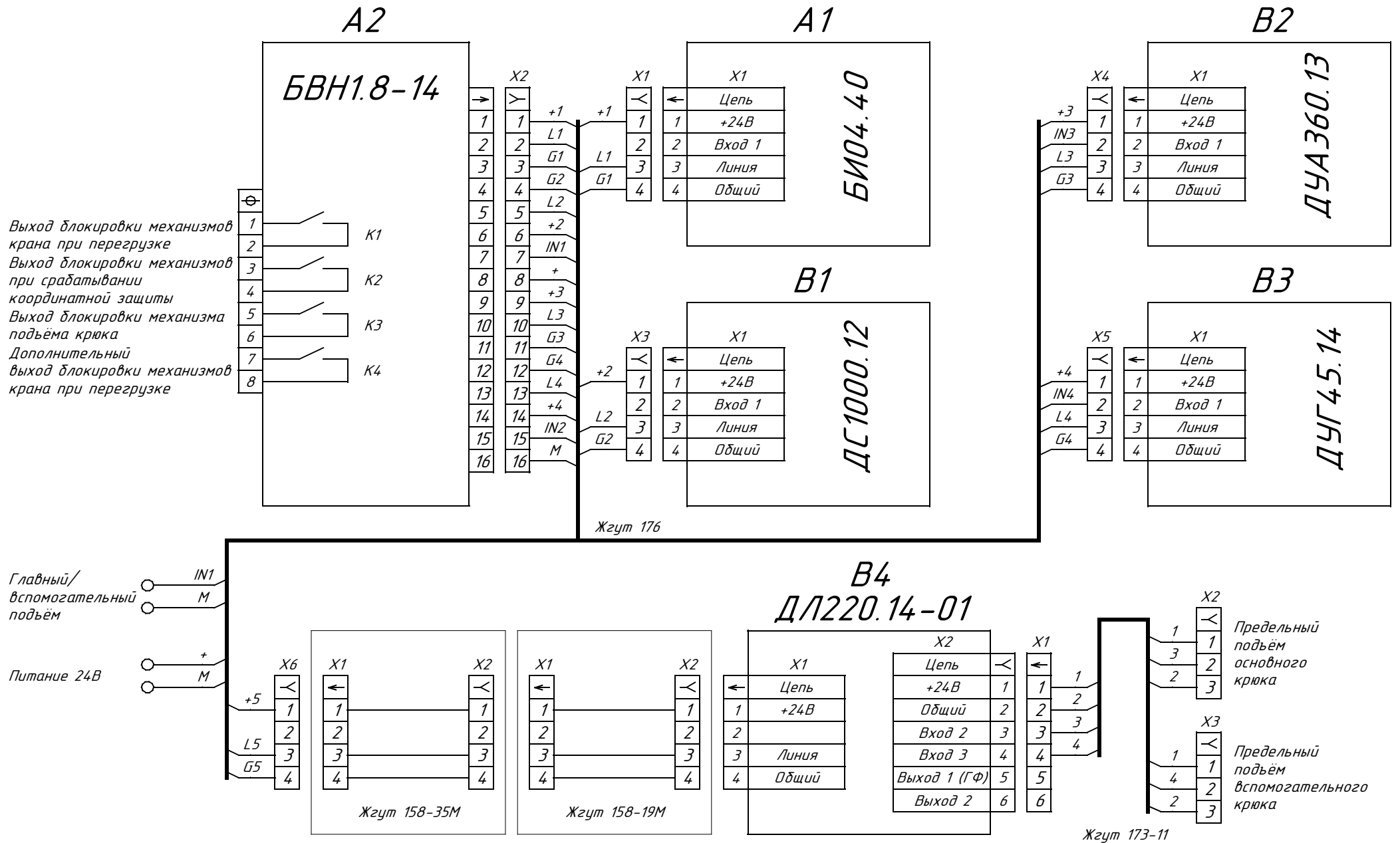
Система безопасности ОГМ240-30.1А-BBB-027.СС Схема электрическая принципиальная
