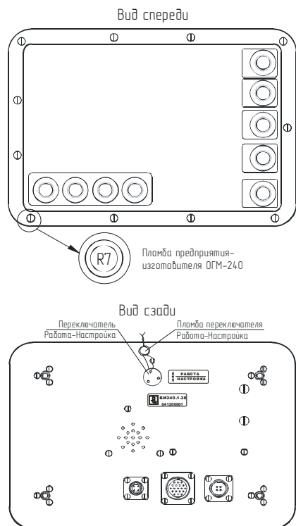
Рисунок 1 — Расположение пломб на блоке индикации
