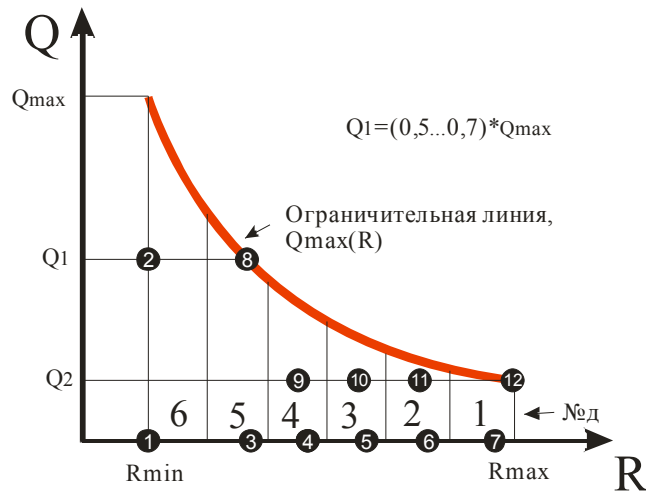
Рисунок 2 — Иллюстрация настройки показаний массы груза
